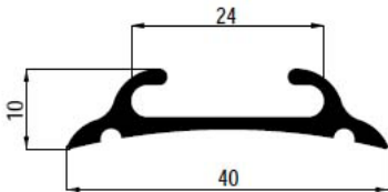
Stootlijst 50 SW (zacht) 1301 400-000 1301 400-011 TZ
