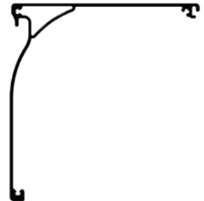
Alu bovenkap 125 mm 6297 920-...
