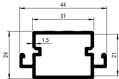
Alu middenprofiel 8000 070-...
