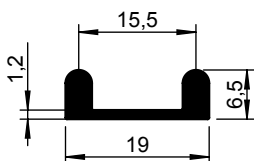
Onderrail (51 ST) 1192 001-000 Brute 1192 001-001 TZ 1192 001-002 Decor. zilver
