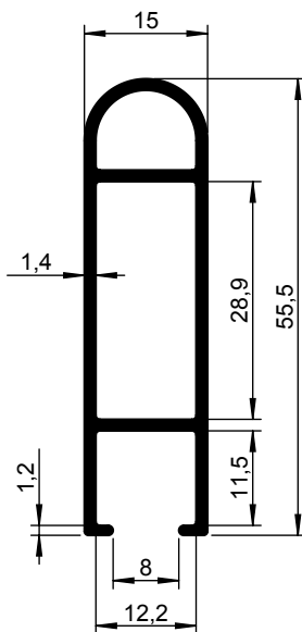
6296 012-000 6000 mm 6296 012-016 TZ 6000 mm
