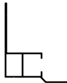
Alu zijgeleider "LHTF" met lip, 60 x 50 mm 6296 802-...
