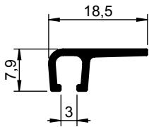
Afsluitprofiel voor borstel Lengte 6000 mm 8000 032-001 TZ 8000 032-006 Wit 8000 032-007 Bruin 8000 032-901 Creme wit
