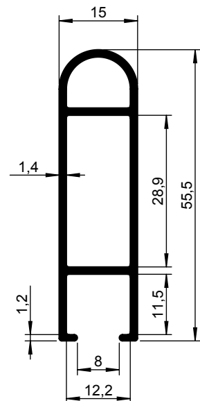
Alu profiel 55x15mm 6296 013-...
