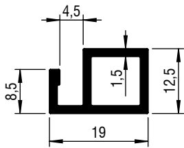
Alu horprofiel 19 mm 8000 005-...
