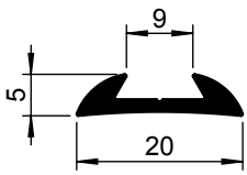
Sierlijst 1119 000-000 1119 000-011 TZ
