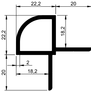
Systeemprofiel afgerond m/2 lippen 1274 630-000 6000 mm 1274 630-001 TZ
