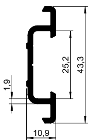
Houderprofiel voor stootrubber 1301 056-000
