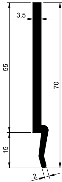
Haak 1274 602-063
