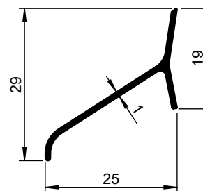
Lekdorpel 1139 000-000 1139 000-001 TZ
