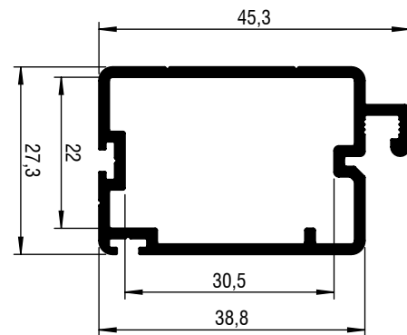
Buitenkader glad met borstelopname 8000 110-...
