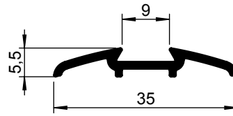
Sierlijst Lengte 4500 mm 1103 351-011 TZ
