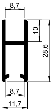
Loopschoen 1192 006-001 TZ
