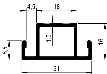
Alu middenprofiel 8000 050-...
