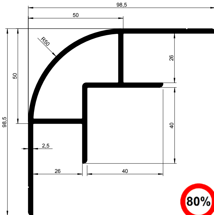
Voorhoekprofiel 1320 180-000 5000 mm 1320 185-000 6000 mm
