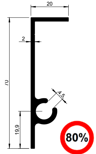
Hoektouwprofiel 1245 700-000
