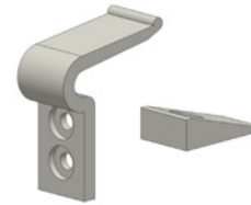
Kunststof spie + klemveer 8002 115-080
