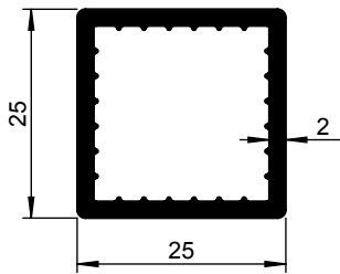
Systeemprofiel zonder lip 1225 025-000 1225 025-010 TZ geanodiseerd
