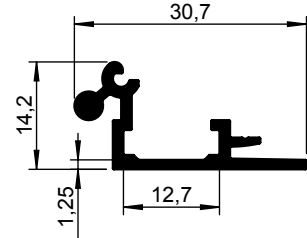
Basisprofiel 32 mm - 6000 mm 1279 050-000
