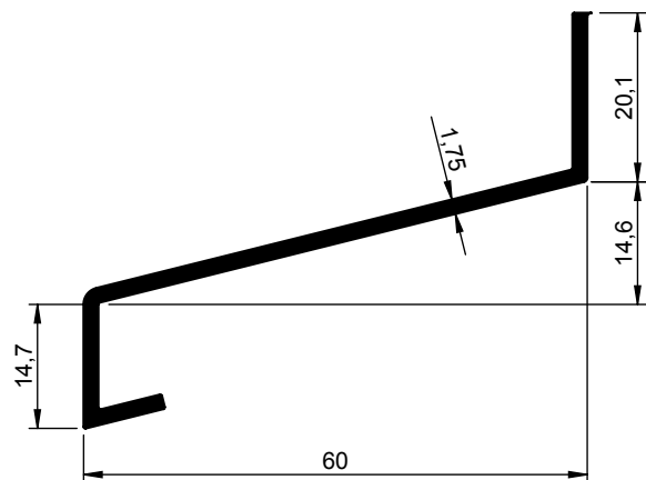
Waterslagprofiel 1144 050-000 1144 050-001 TZ
