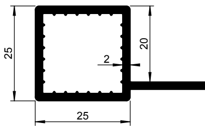
Systeemprofiel met 1 lip 1225 028-000 1225 028-010 TZ geanodiseerd
