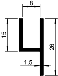
1142 100-000 1142 100-001 TZ
