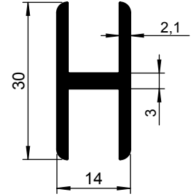
1256 070-000 1256 070-001 TZ
