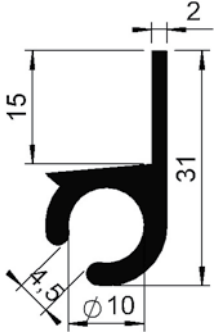
Touwprofiel (zacht) 1240 000-000 1240 000-011 TZ
