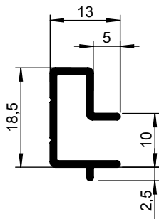
Strokenwandprofiel 1273 500-000
