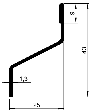
Lekdorpel 1137 000-000 1137 000-001 TZ
