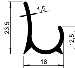
Gootlijst (zacht) 1245 000-000 1245 000-011 TZ
