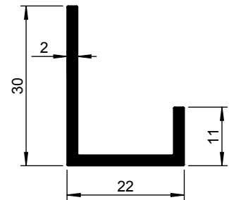
1113 500-000 1113 500-001 TZ
