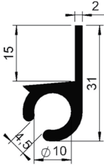
Touwprofiel 1240 000-...
