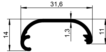
Wissellijstprofiel 32 mm - 6000 mm 1279 052-000 1279 052-001 TZ
