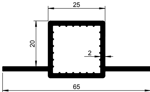
Systeemprofiel met 2 lippen horizontaal 1225 031-000 1225 031-010 TZ geanodiseerd
