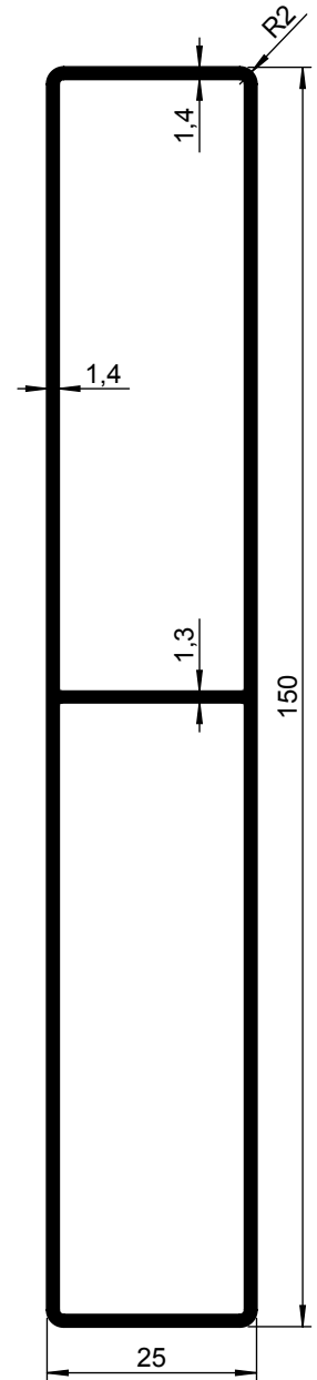
Eindkap (2x) 75 x 25 mm 1320 085-000 6000 mm 1320 085-011 TZ 1320 086-000 6500 mm
