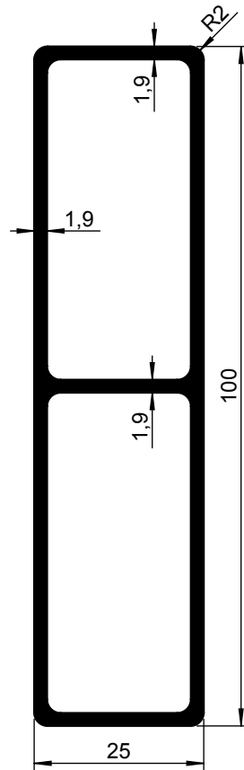
Eindkap 100 x 25 mm 1320 000-000 6600 mm 1320 000-011 TZ 1320 002-000 7500 mm 1320 002-011 TZ
