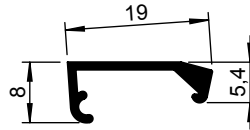
Wissellijstprofiel 18 mm: 6000 mm 1279 002-000 1279 002-001 TZ
