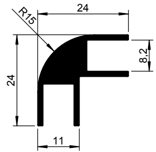
Hoekprofiel afgerond 1198 000-000 1198 000-001 TZ 1198 000-002 DZ
