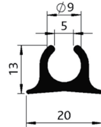
Tentrailprofiel 1305 081-...
