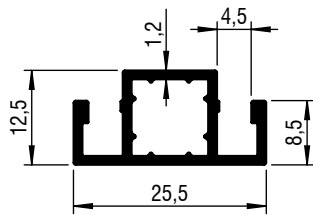
Alu middenprofiel 8000 010-...
