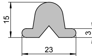
Stootrubber voor 1301 400-000 2460 010-000
