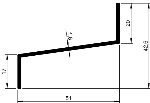
Waterslagprofiel 1144 025-000
