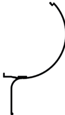
Alu onderkap 95 mm rond met lip 6296 372-...
