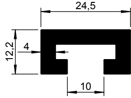
1185 000-000 1185 000-001 TZ 1185 000-002 DZ
