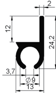
Touwprofiel 1240 100-...
