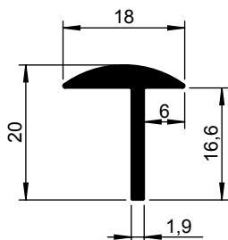
1102 200-000 1102 200-001 TZ
