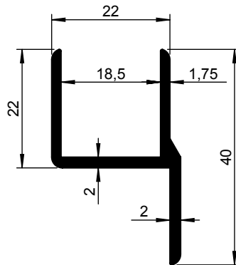
1305 310-000 1305 310-011 TZ
