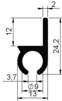
Touwprofiel (zacht) 1240 100-000 1240 100-011 TZ
