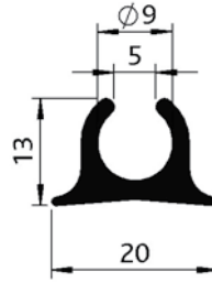
Tentrailprofiel (zacht) 1305 080-000 1305 080-011 TZ
