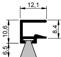
Stofborstelprofiel geanodiseerd 3543 007-000 (incl. borstel 6,5 mm)
