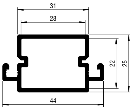
Alu tussenkader glad 8000 106-...
