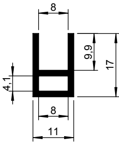
Alu voorzetraamprofiel 8100 002-...
