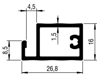
Alu hordeur 26 mm 8000 045-...
