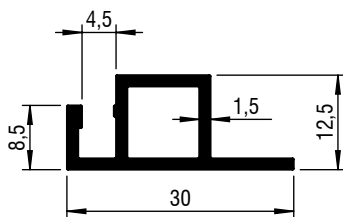
Alu horprofiel 30 mm 8000 040-...
