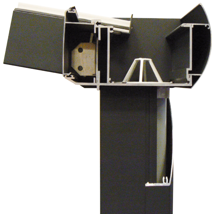
Doorsnede Piazza® gootprofiel
