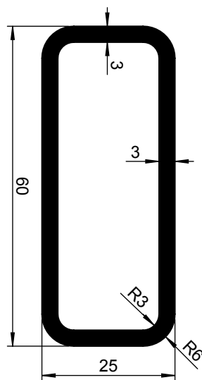
0102 656-000 6000 mm 0102 656-011 TZ
