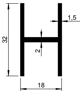
1256 064-000 1256 064-011 TZ
