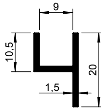
1142 050-000 1142 050-001 TZ
