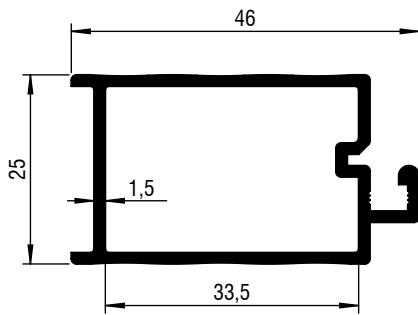
Alu horprofiel 46 x 25 mm 8000 065-...
