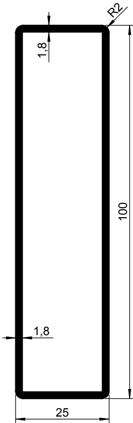
Eindkap 100 x 25 mm 1317 160-000 6600 mm 1317 160-011 TZ 1317 150-000 7500 mm 1317 150-011 TZ
