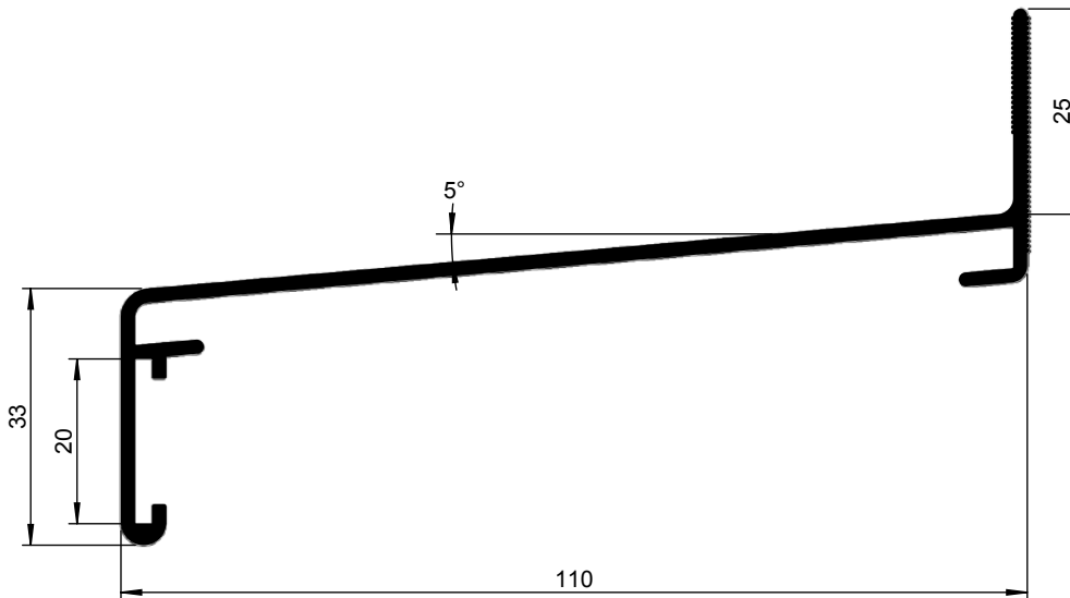
Waterslagprofiel - lengte 6000 mm 1144 110-000 Gemoffeld op aanvraag
