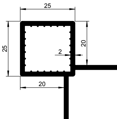
Systeemprofiel met 2 lippen hoek 90° 1225 034-000 1225 034-010 TZ geanodiseerd
