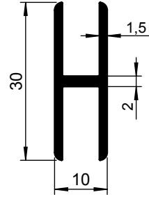
1256 062-000 1256 062-001 TZ
