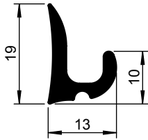
Gootlijst (zacht) 1305 115-000 1305 115-011 TZ
