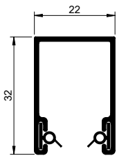
Zijgeleider TF 3105 000
