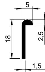
1128 000-000 1128 000-001 TZ
