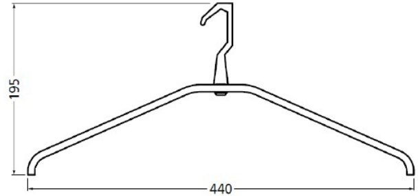
Kledinghanger zelfrichtend 3670 120-002
