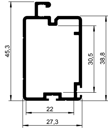
Buitenkader glad met borstelopname 8000 110-...
