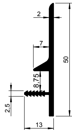
1180 500-001 TZ Lengte 6000 mm
