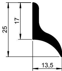
Vleugellijst (zacht) 1305 130-000 1305 130-011 TZ
