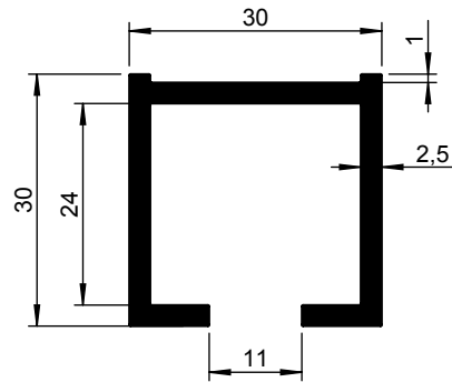
6296 301-000 7500 mm 6296 301-016 TZ 7500 mm
