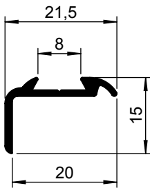
Caravan hoeklijst 50 SW (zacht) 1305 000-000 1305 000-011 TZ
