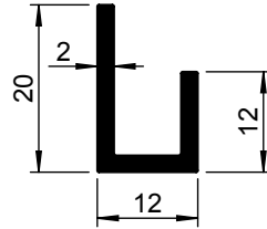
1113 600-000 1113 600-001 TZ
