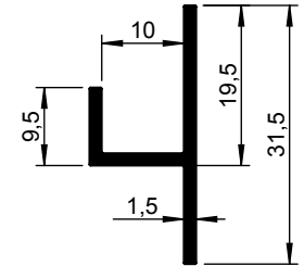
1256 050-000 1256 050-001 TZ
