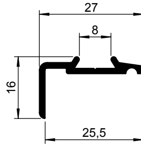
Caravan hoeklijst 50 SW (zacht) 1305 015-000 1305 015-011 TZ
