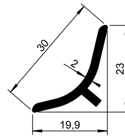
Plintprofiel (zacht) 1305 040-000 1305 040-001 TZ
