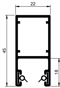
Zijgeleider H17 1102 000
