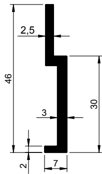
Haakprofiel 1274 600-000 6000 mm
