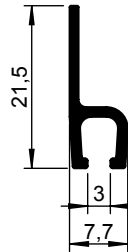
Afsluitprofiel voor borstel Lengte 6000 mm 8000 033-001 TZ 8000 033-006 Wit 8000 033-007 Bruin 8000 033-901 Creme wit
