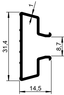
Strokenwandprofiel dubbel 1273 505-000
