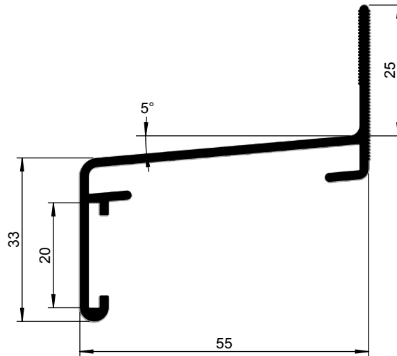
Waterslagprofiel - lengte 6000 mm 1144 055-000 Gemoffeld op aanvraag
