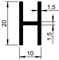
1256 060-000 1256 060-001 TZ
