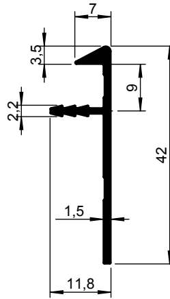
1181 042-000 1181 042-001 TZ
