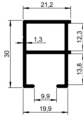
6296 658-000 7000 mm 6296 658-016 TZ 7000 mm
