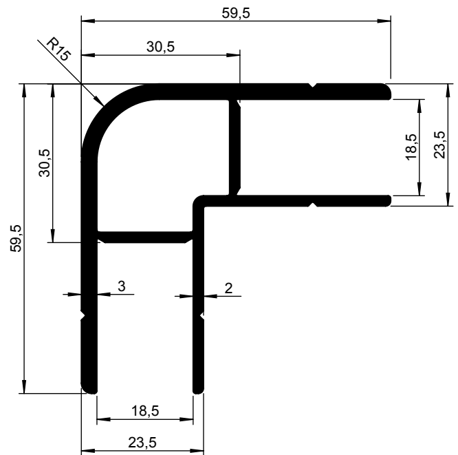
Hoekverbindingsprofiel 1320 900-000 7000 mm 1320 900-011 TZ 7000 mm
