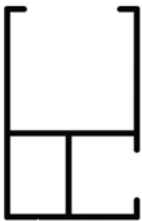
Alu klik-zijgeleider 47 5 x 30 mm 6296 660-...
