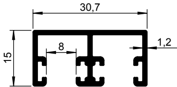
Dubbel U-profiel (bovenrail) 1192 008-000 Brute 1192 008-001 TZ 1192 008-002 Decoratief zilver 1192 008-010 TZ (geboord/verzonken)
