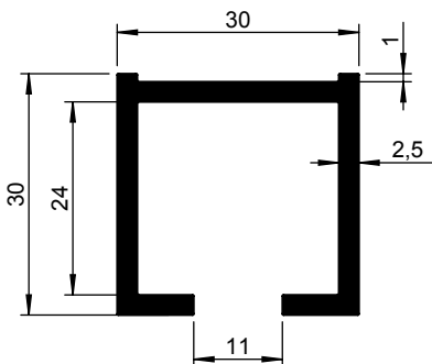
Alu geleiderprofiel 30x30x30x2,5 mm 6296 301-...
