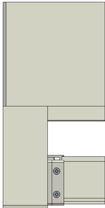
Achteraanzicht
