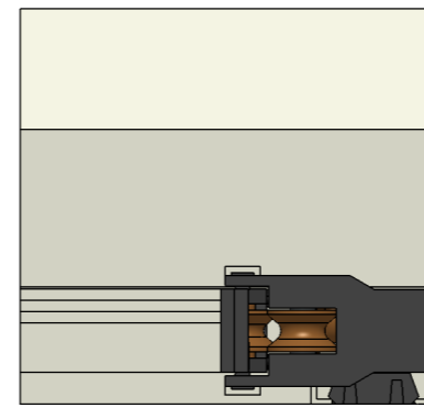
Onderaanzicht
