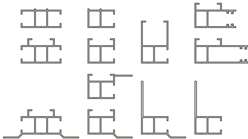
Zijgeleiders
