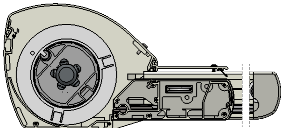
Doorsnede
