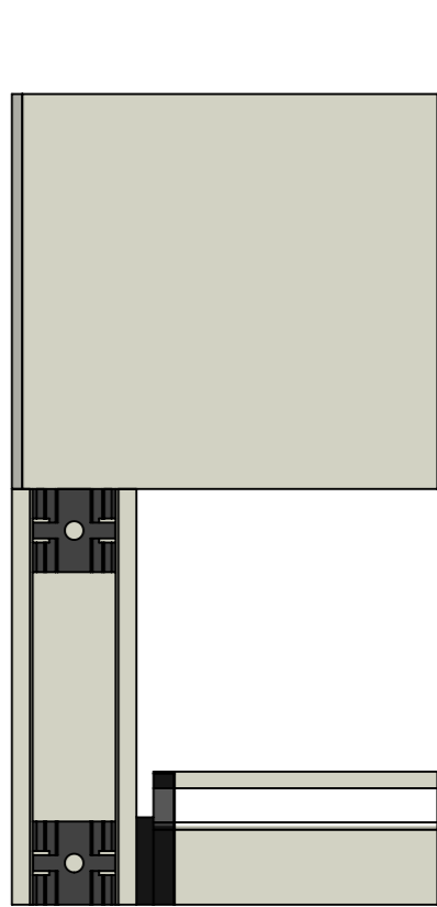
Achteraanzicht
