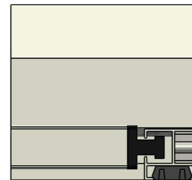
Onderaanzicht
